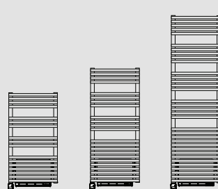
TLN050-050IFS TLNO-050-050-IFS TLN075-050IFS TLNO-050-050-IFS TLN100-050IFS
